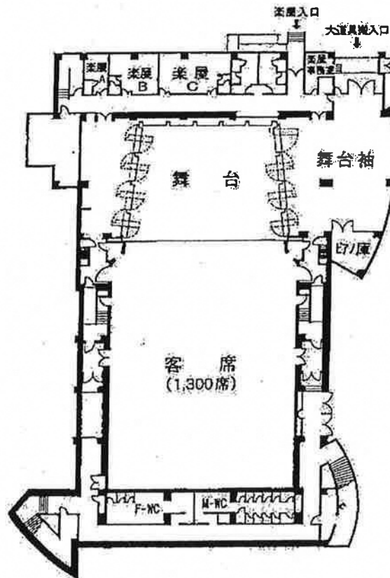
地下平面図
